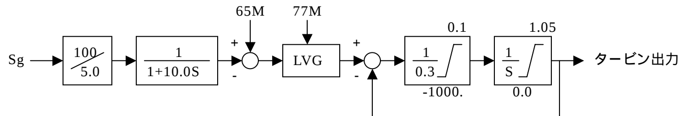
( b ) 水力機用モデル 1 ( L P T = 3 )
