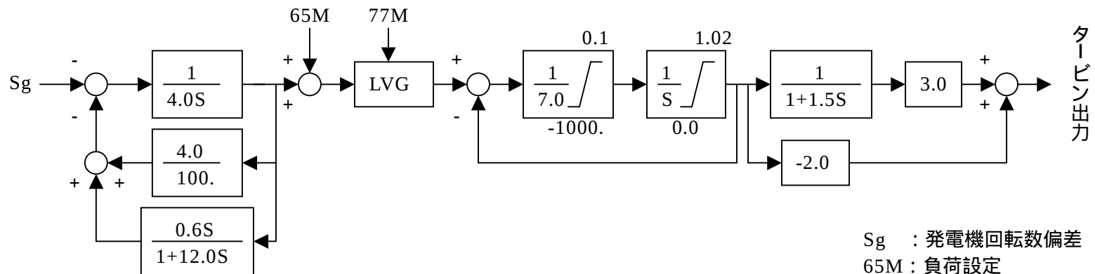
( C ) 水力機用モデル 2 ( L P T = 4 )
