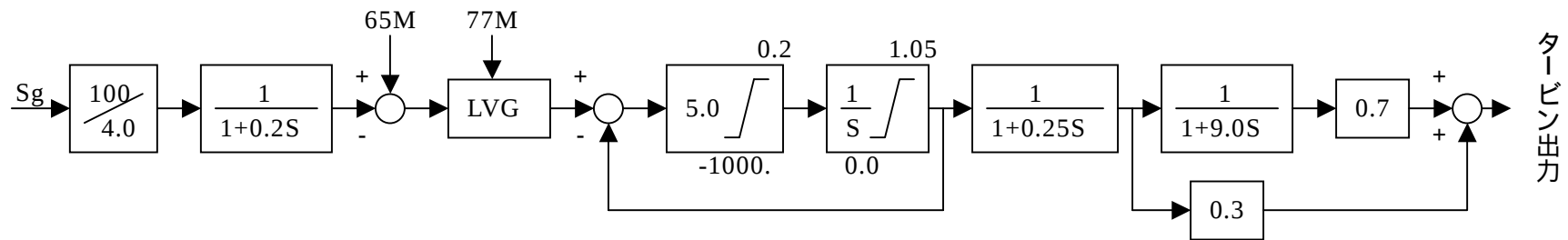
( a ) 火力・原子力機用モデル ( L P T = 1 )
