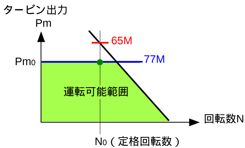
付1.4図 ロードリミット(L.L.)運転
