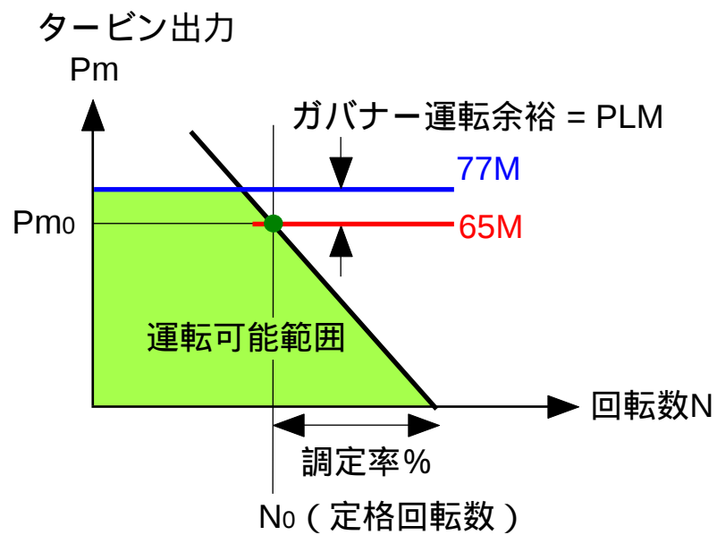
付1.3図 ガバナーフリー(G.F.)運転
