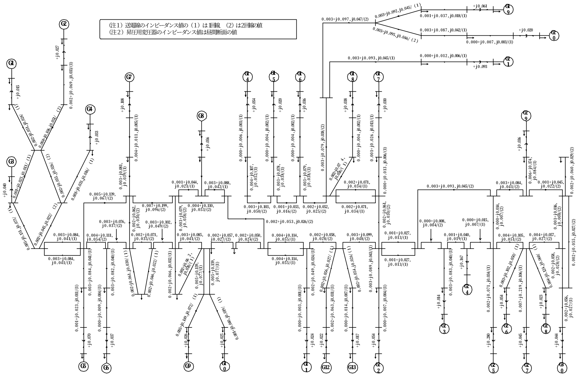
4.23図 電気学会WE S T 3 0機系統モデル インピーダンスマップ (1,000MVAベースpu値)
