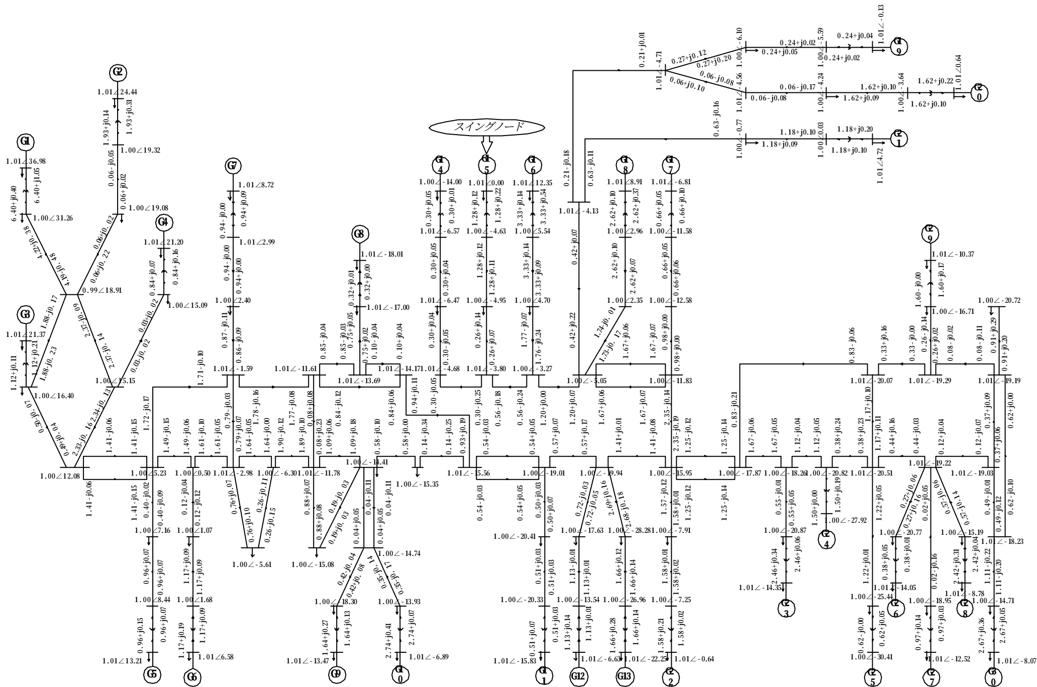
4.24図(b) 電気学会WEST30機系統モデル 潮流図（夜間断面）
