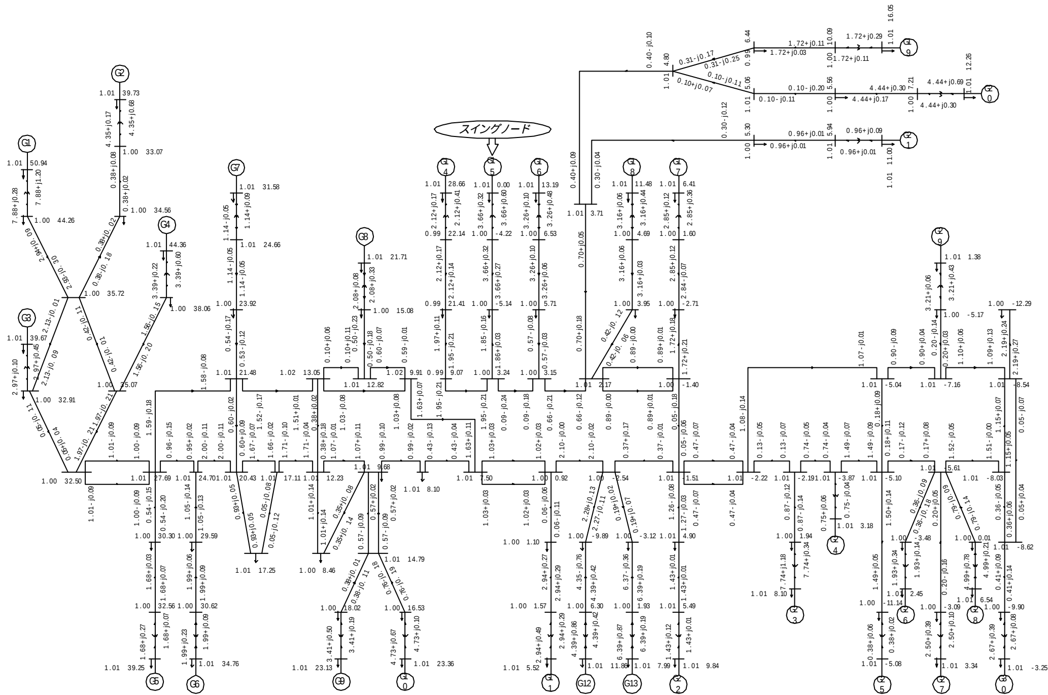
4.24図(a) 電気学会WEST30機系統モデル 潮流図 (昼間断面)
