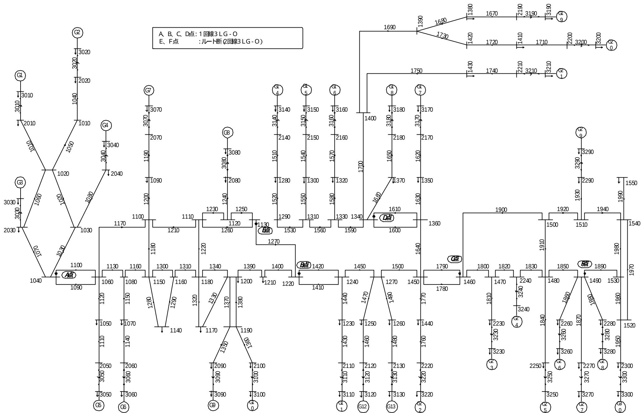
4.22図 電気学会WE S T 3 0機系統モデル 系統図(ノード番号、ブランチ番号、事故点含む)
